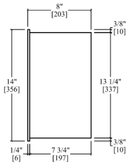
'B' View(Side)
