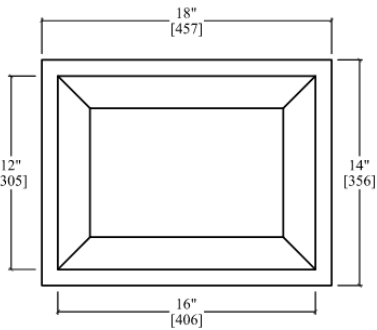
'A' View(front)
